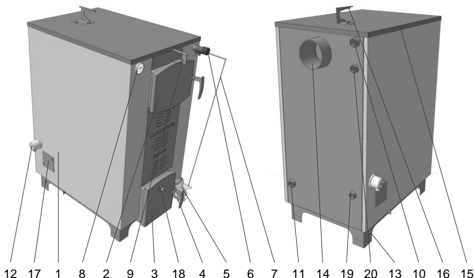
Рис. 1. Конструкция котла модельного ряда «Суворов Ультра»
