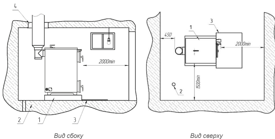
1 — основание, 2 — дренажное отверстие, 3 — лист металла, 4 — песочница
