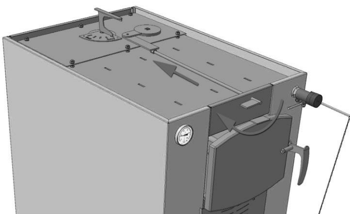
Рис. 8. Чистка теплообменной полости котла
