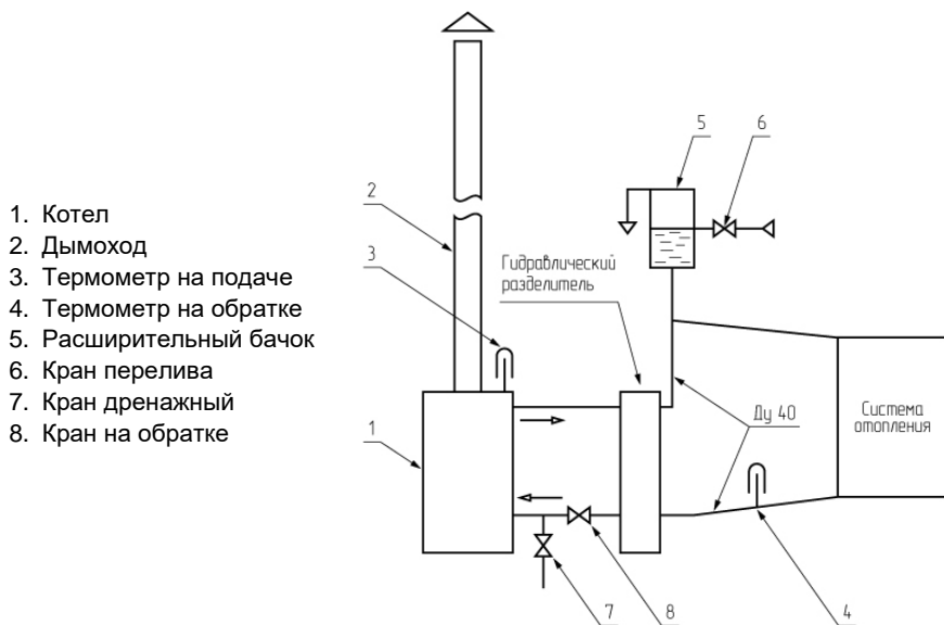
Рис. 4. Подключение к открытой системе отопления с естественной циркуляцией
