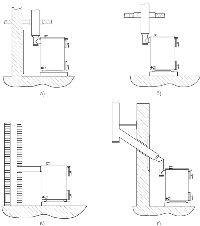
Рис. 3. Рекомендуемые схемы подключения котла к системе дымоотведения
