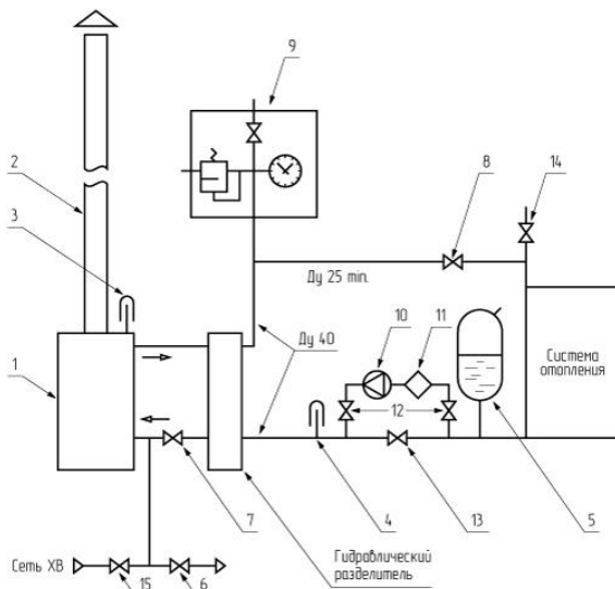
Рис. 6. Подключение к закрытой системе отопления
