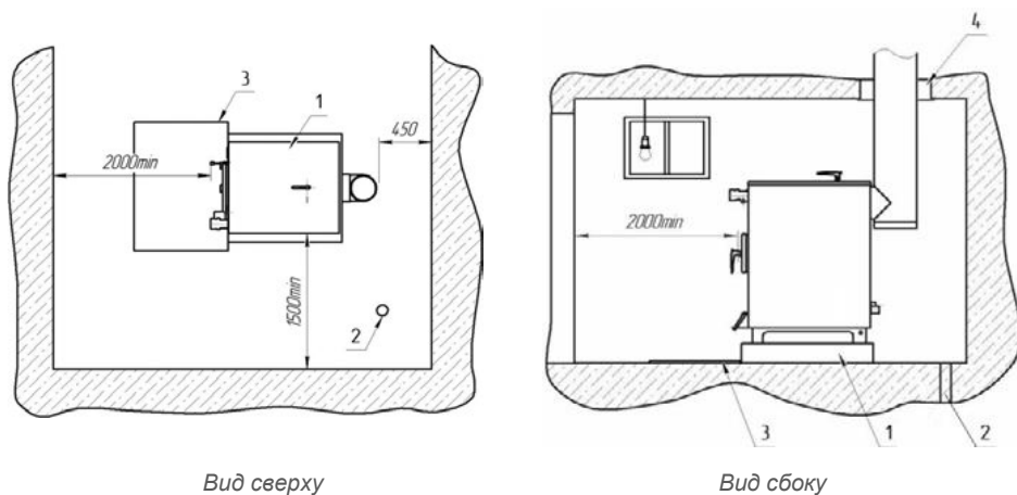
Рис. 2. Условия монтажа котла «Суворов Эко»
