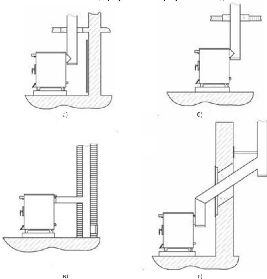
Рис. 3. Рекомендуемые схемы подключения котла к системе дымоотведения
